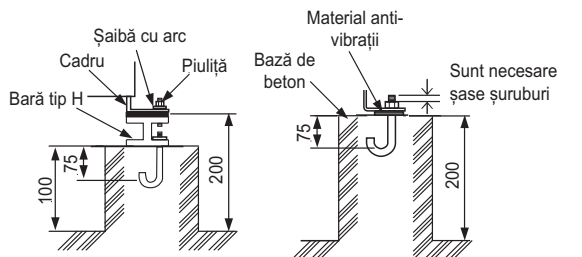
Metoda de montare a bolțurilor pentru fundație
