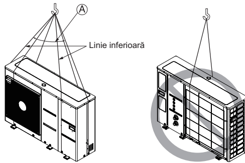
A unghi de 40° sau mai mic
