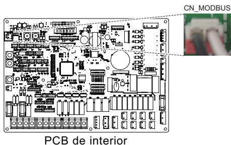
PCB de interior
