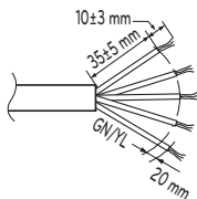
Pentru un sistem trifazic
