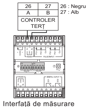
Interfață de măsurare
