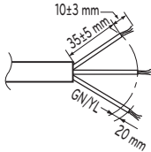
Pentru un sistem monofazic
